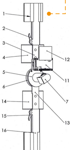
Vista isométrica derecha del transductor háptico de movimientos flexión-extensión.
