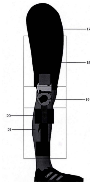
Vista frontal del transductor háptico de movimientos flexión-extensión en rodilla colocado al usuario.
