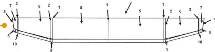
Vista lateral del ala morfológica en su posición inicial, sin articulación.
