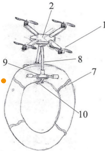
Vista isométrica del vehículo
